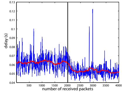
(d) Delay behavior when D_{\max} changes from 1 s to 60 ms
