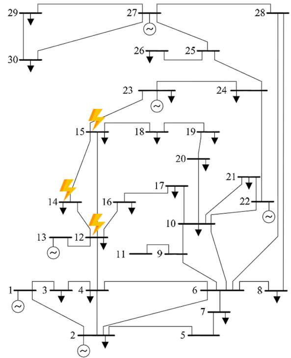
Fig. 4. IEEE 30-bus test case [35].
